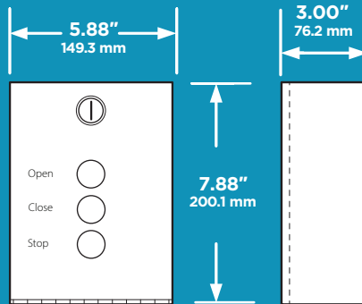
1200-006 3-Button Interior/Exterior
